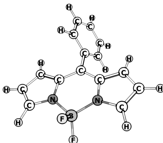
Рис. 1: Модель молекулы 8-фенил-BODIPY
